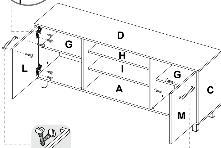
Manija/ Handle
