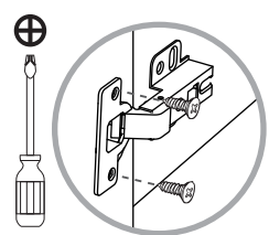
Ajuste de las bisagras Hinge adjustment
