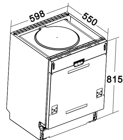
Dimensión de instalación Medidas en mm
